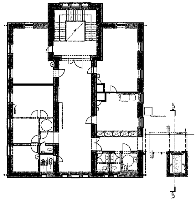
Alaprajz - Emelet M=1:300
