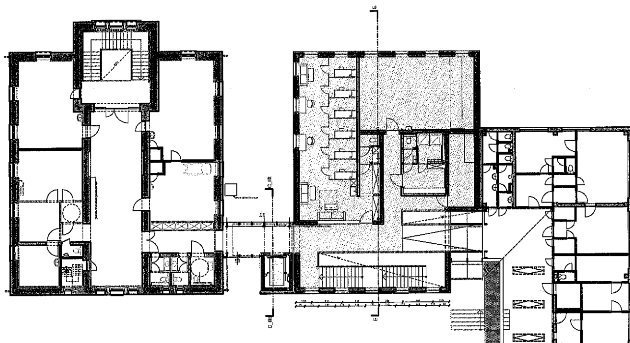
Alaprajz - Emelet M=1:300
