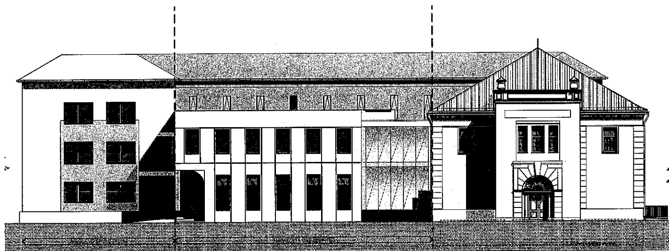
Homlokzat- Szilfákálja út felőli M=1:300
